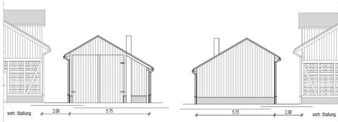
Nord-Ansicht
